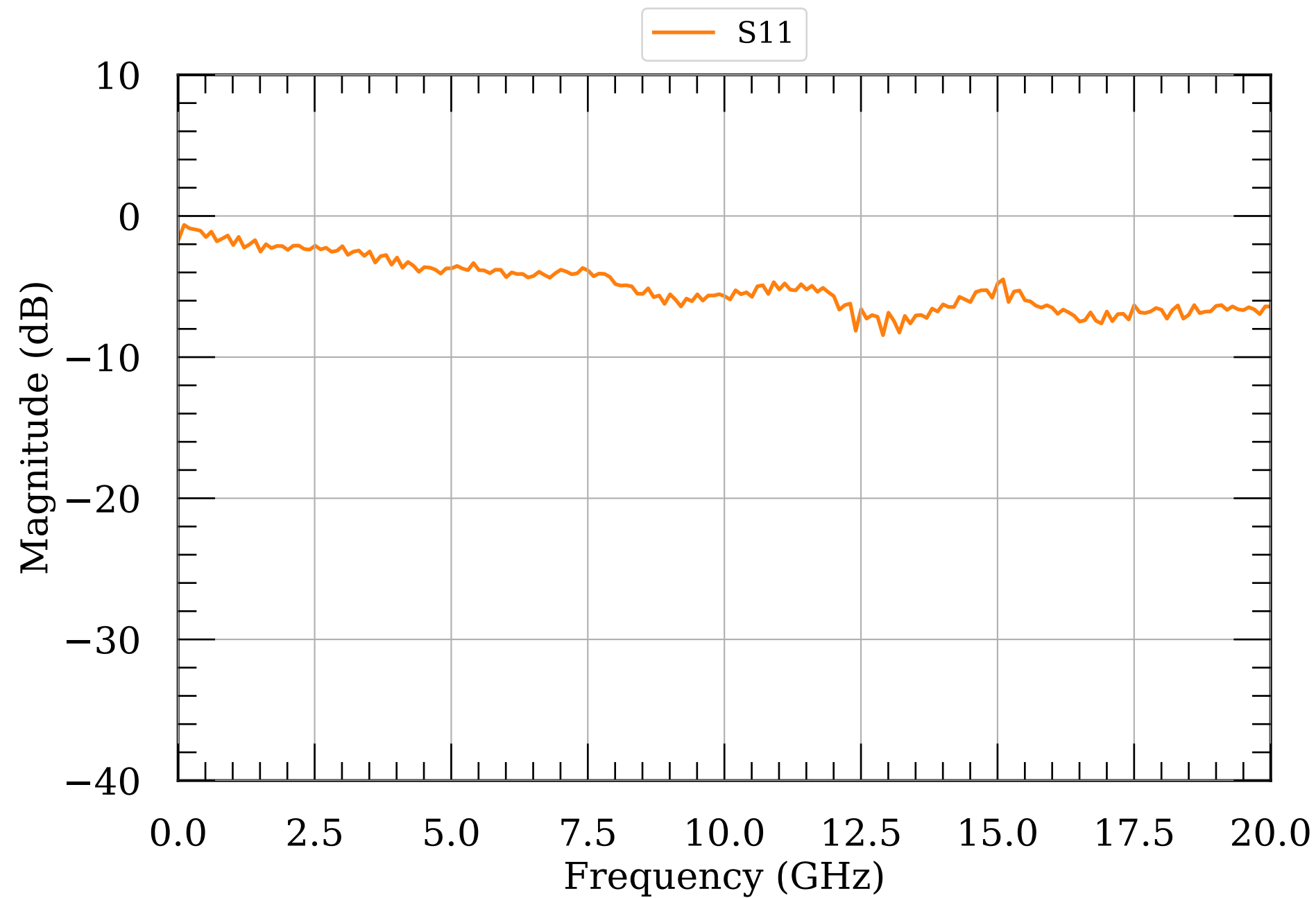
LNA S-params module023
